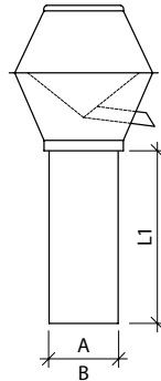
Regenhut eckig mit Standrohr
