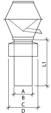
Regenhut eckig mit Regenkragen
