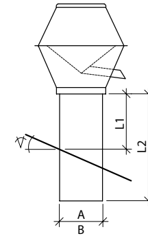
Regenhut eckig mit Tablett (Steildach \triangle )
