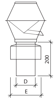
Regenhut rund mit Regenkragen und Steckmuffe
