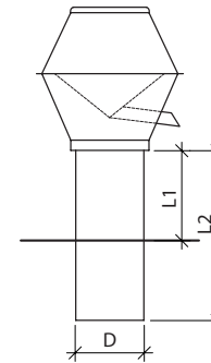
Regenhut rund mit Tablett (Flachdach 0°)
