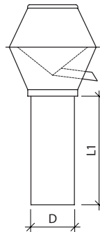
Regenhut rund mit Standrohr
