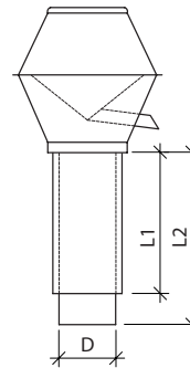
Regenhut rund doppelwandig
